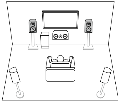
5.1 ch (Bi-Amping (Front)) ( →p31)
