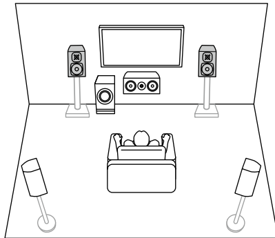
5.1 ch (Bi-Amping (Front)) ( →p27)
