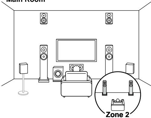
5.1.2 ch + ZONE 2 (→p28)
